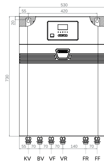
Tilslutningsskitse, højrevendt
