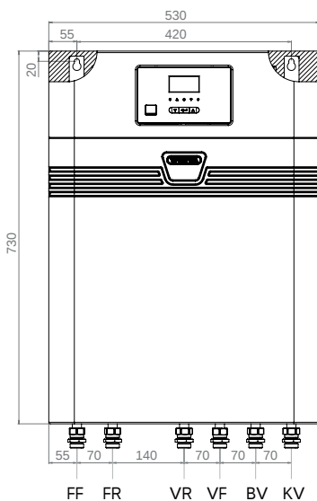
Tilslutningsskitse, venstrevendt
